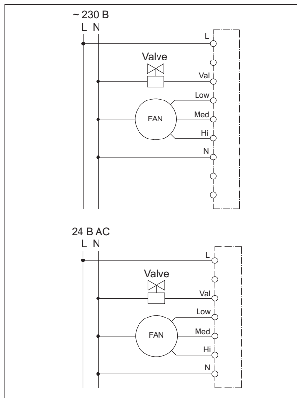
Схема подключения
